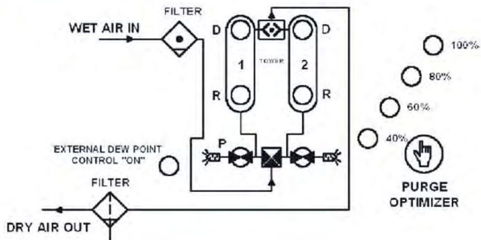
Control Panel DS 31-200
